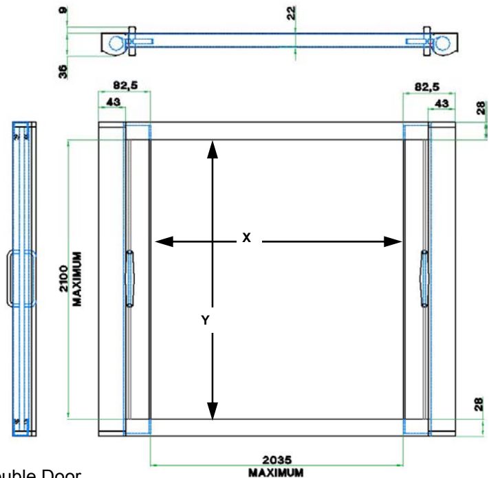
Double Door
